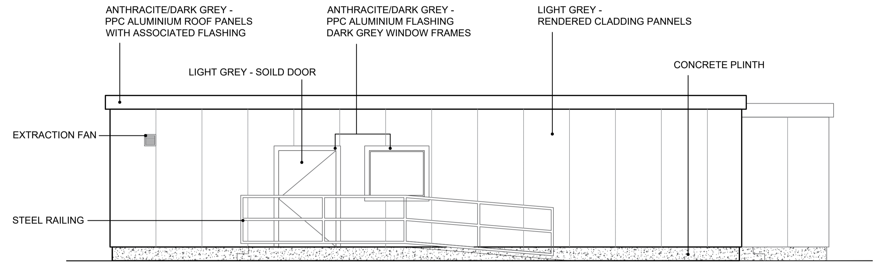
ELEVATION B
